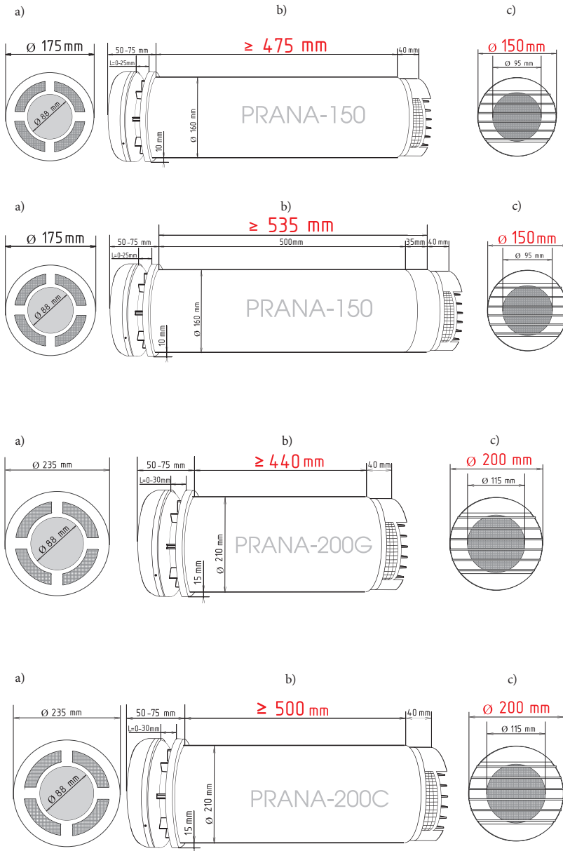
Poza 4. Dimensiunile și schițele recuperatoarelor «PRANA-150», «PRANA-200G», «PRANA-200C»: a) grilla de ventilare și admisie din încăpere; b) unitatea de lucru (lateral); c) grilla de ventilare și admisie din exterior.
