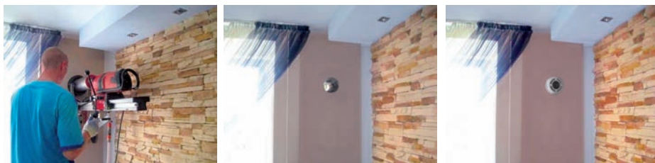
Poza 6. Exemplu de montare recuperator «PRANA-150», «PRANA-200G», «PRANA-200C».
