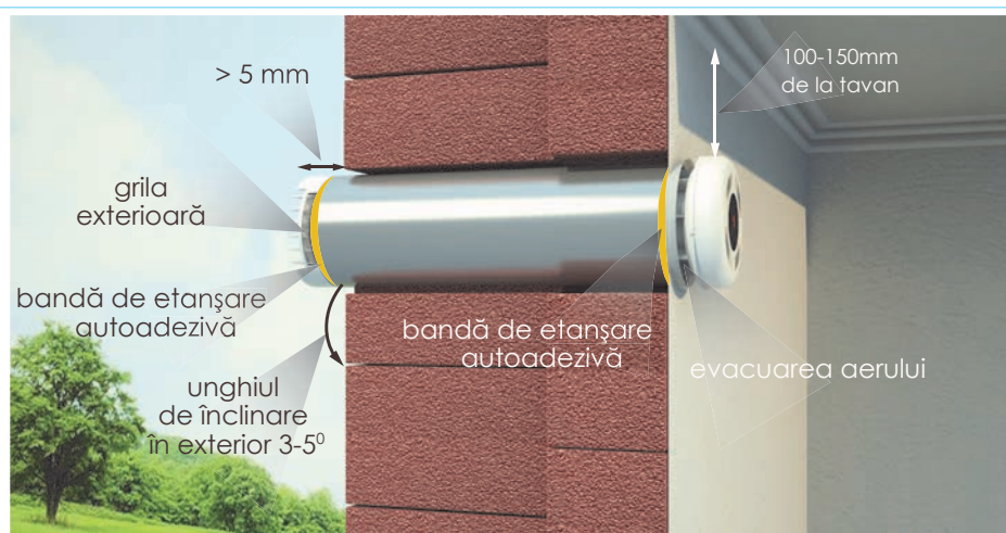
Poza 5. Schema de montare a recuperatorului în perete .
