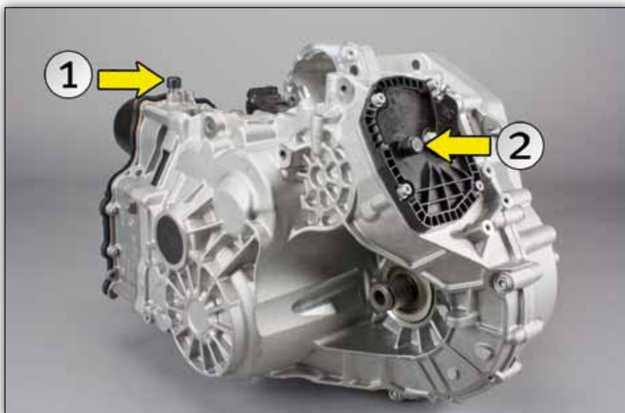
Fig. 1: Cutie de viteze automată cu capace de aerisire pentru unitatea mecatronică (1) și cutia de viteze (2).
