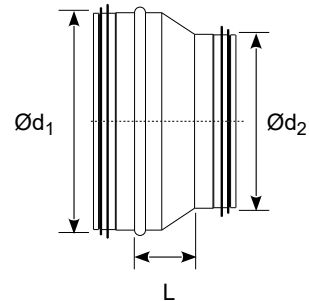
Reductie presata
