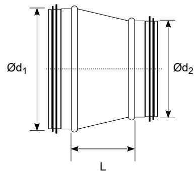
Reductie faltuita
