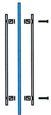
schema montaggio maniglia
