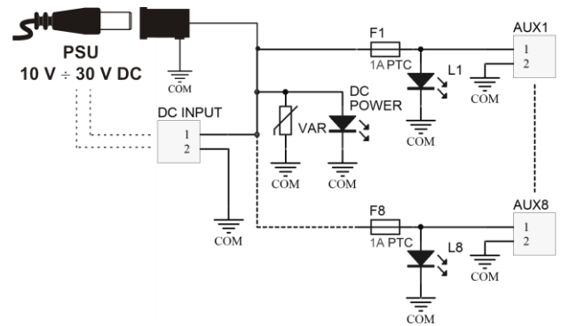
Fig.2. Block diagram.
