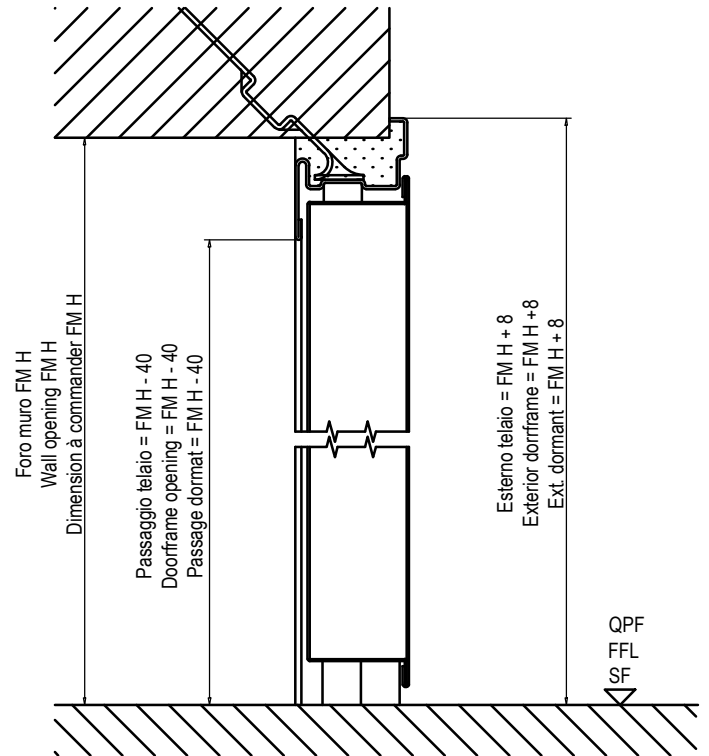
Sezione verticale Vertical cross section Coupe vertical
