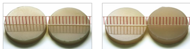
Compozitul Mosaic lustruit înainte de periaj | Compozitul Mosaic după 10.000 cicluri de periaj | Alt compozit lustruit înainte de periaj | Alt compozit după 10.000 cicluri de periaj
