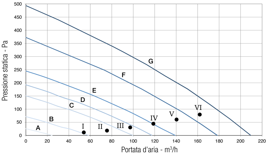
Fig. 6.a Curva di immissione in accordo al Regolamento 1253/2014 (ErP).
