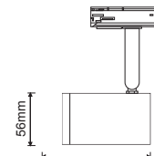
Μονοφασικά σποτ ράγας 1 phase track luminaires GU10
