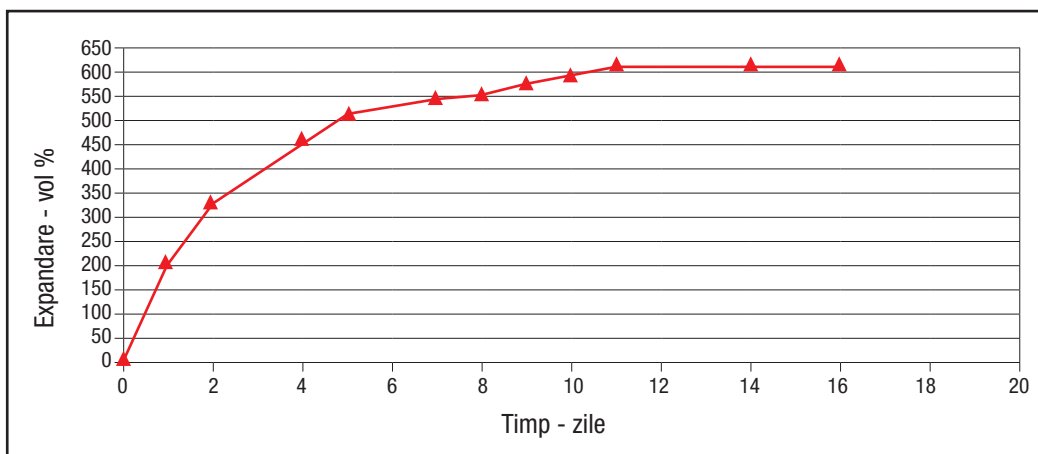
Fig. 1: graficul expandării volumetrică a Idrostop Soft în apa distilată la +25°C în conformitate cu norma JIS K6258:1993
